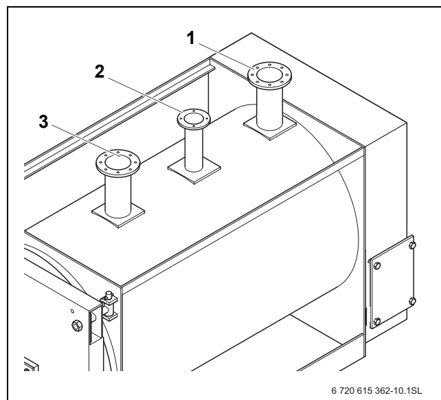
10. pav. Šildymo katilas "Logano" nuo 1400 kW iki 3500 kW
