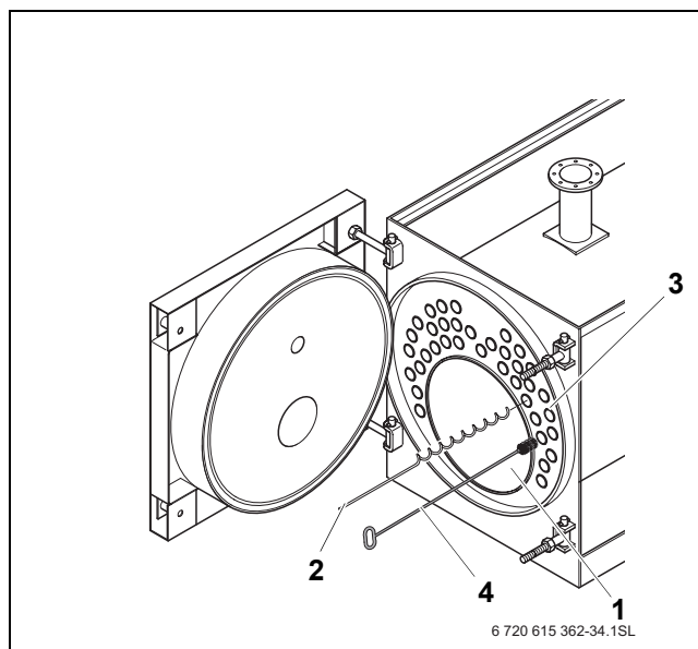
34. pav. Degimo paviršių valymas
