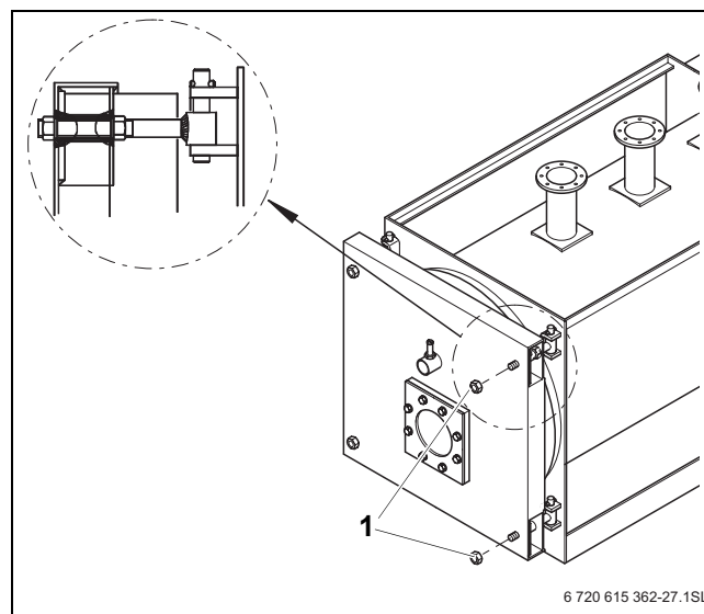
27. pav. Degiklio durelių atidarymas
