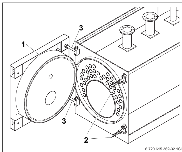
32. pav. Degiklio durelių atidarymas
