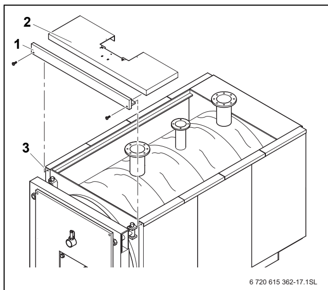
17. pav. Priekinio katilo gaubto montavimas
