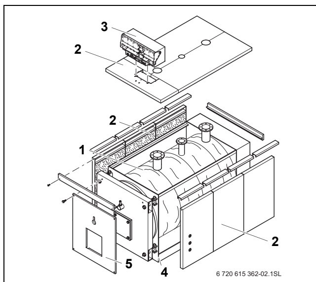
2. pav. Skystojo kuro / dujų specialusis šildymo katilas "Logano" 1400 kW-3500 kW
