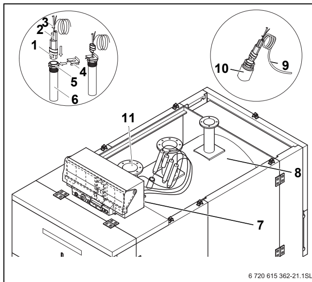
21. pav. Temperatūros jutiklių komplekto montavimas
