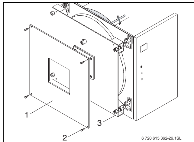
26. pav. Skersinių dangčių montavimas
