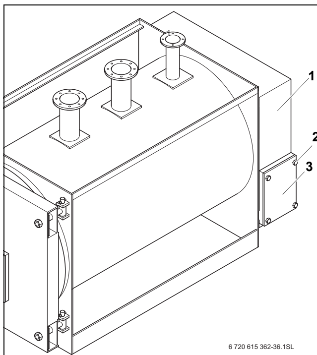
36. pav. Valymo angų dangtelių nuėmimas
