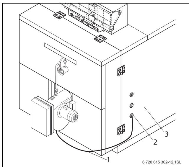
12. pav. Degiklio kabelio montavimas
