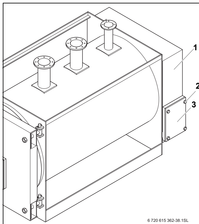
38. pav. Valymo dangtelio uždėjimas
