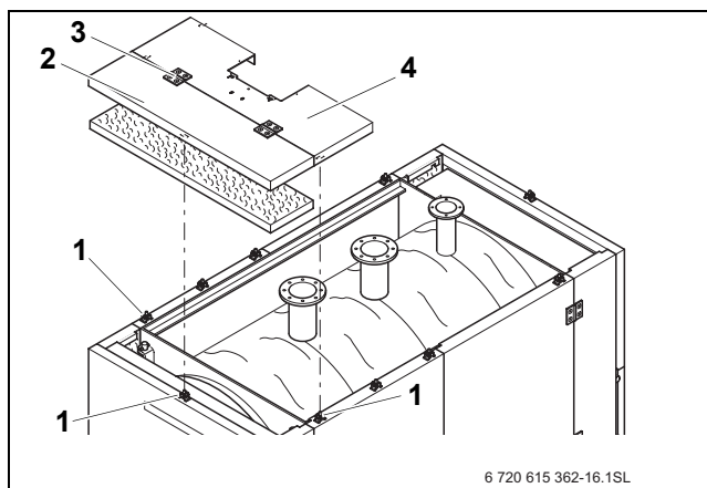
16. pav. Priekinio katilo gaubto montavimas
