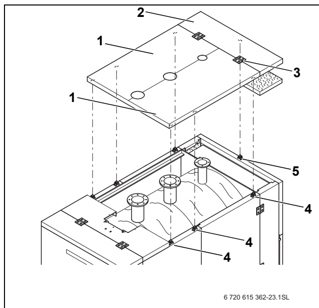
23. pav. Katilo gaubtų montavimas
