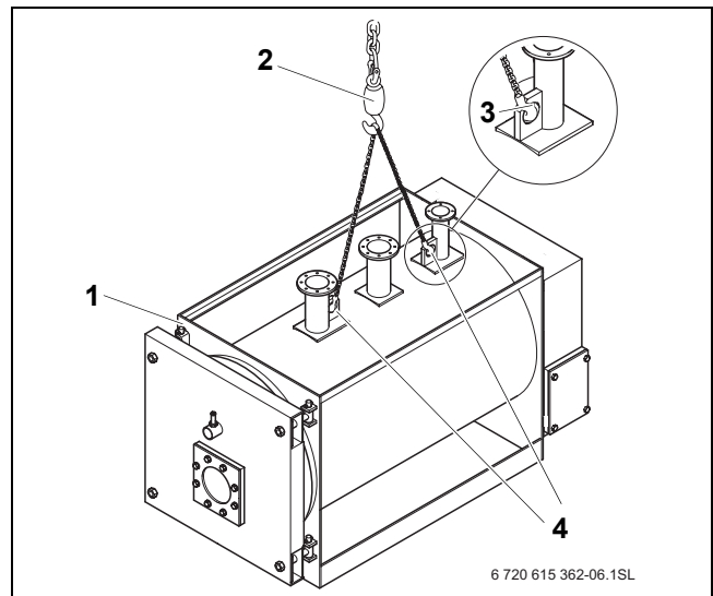
6. pav. Katilo korpuso kėlimas kranu
