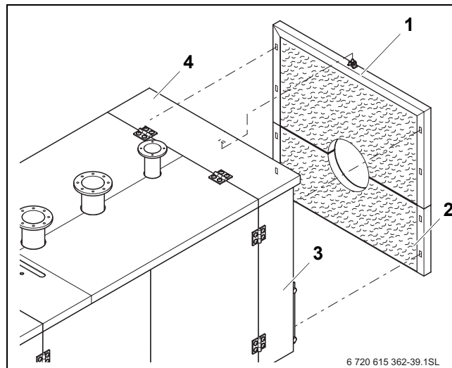
39. pav. Užpakalinės sienelės dalių montavimas
