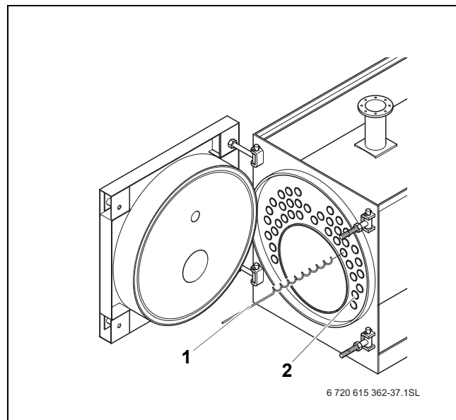
37. pav. Suktukų padėties koregavimas
