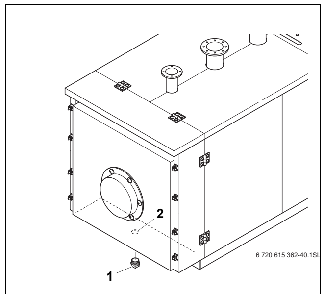
40. pav. Nutekėjimo vamzdelio atidarymas / uždarymas
