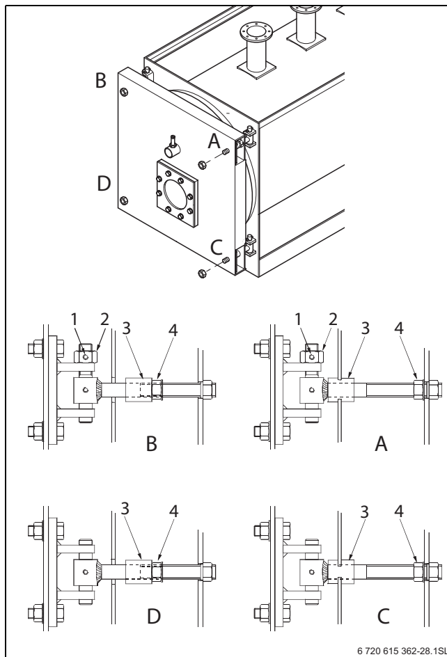
28. pav. Degiklio durelių atidarymas
